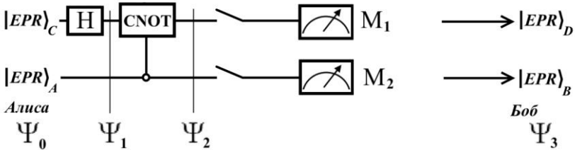
Рис.2. Установка для телепортации запутанности
